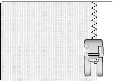
Nastavenie pre trojstupňový kľukatý steh
