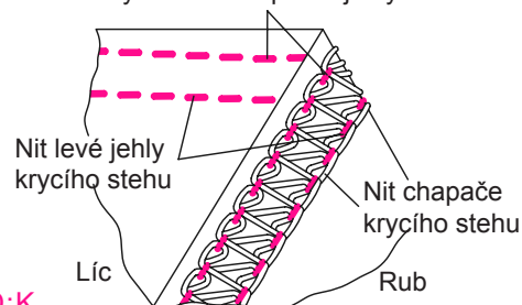
Krycí steh nitě pravé jehly
