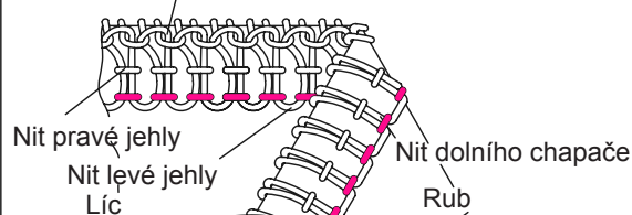
Nit horního chapače
