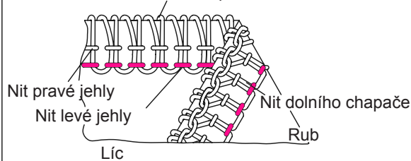
Nit horního chapače
