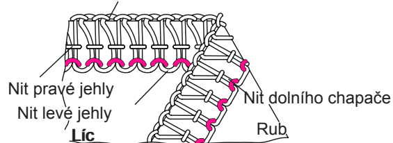
Nit horního chapače
